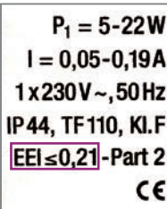
Typenschild
